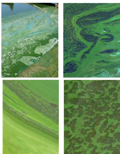
Aspect possible d'une efflorescence de cyanobactéries
