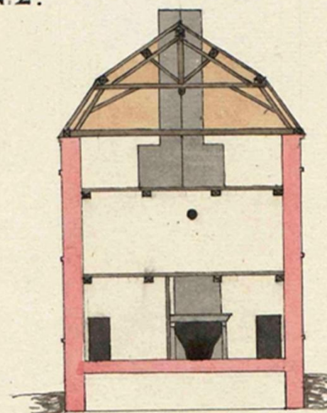
Coupe transversale.
