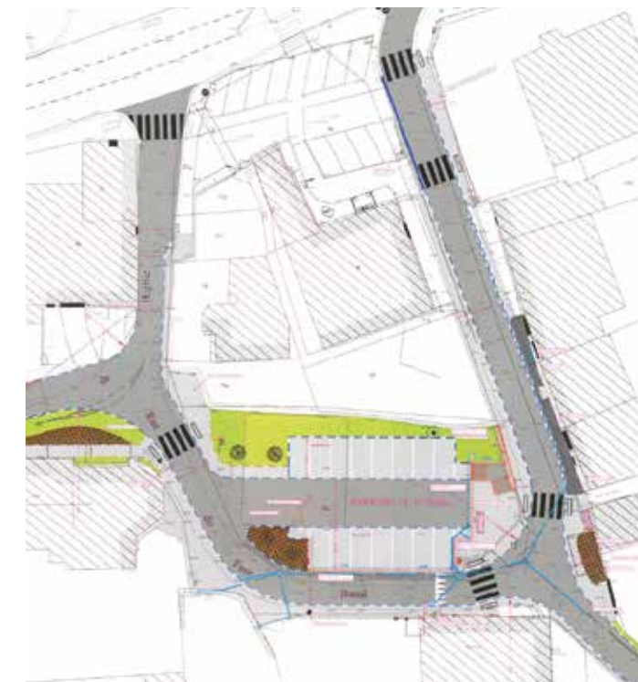
Aménagement d'un parking fermé
