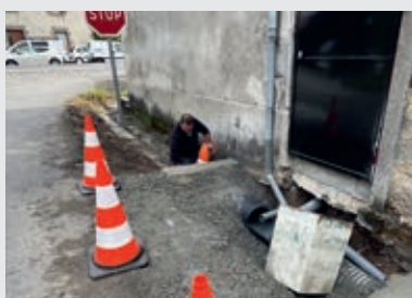
Réfection assainissement La Bouteille
