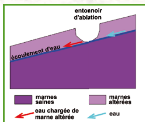
Fig. 5 : Formation des entonnoirs d'ablation sur un versant marneux.
