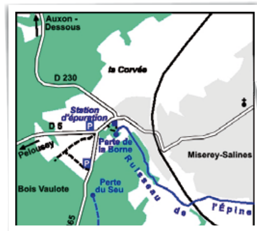
Fig. 2 : Localisation des pertes de la Borne à Miserey
