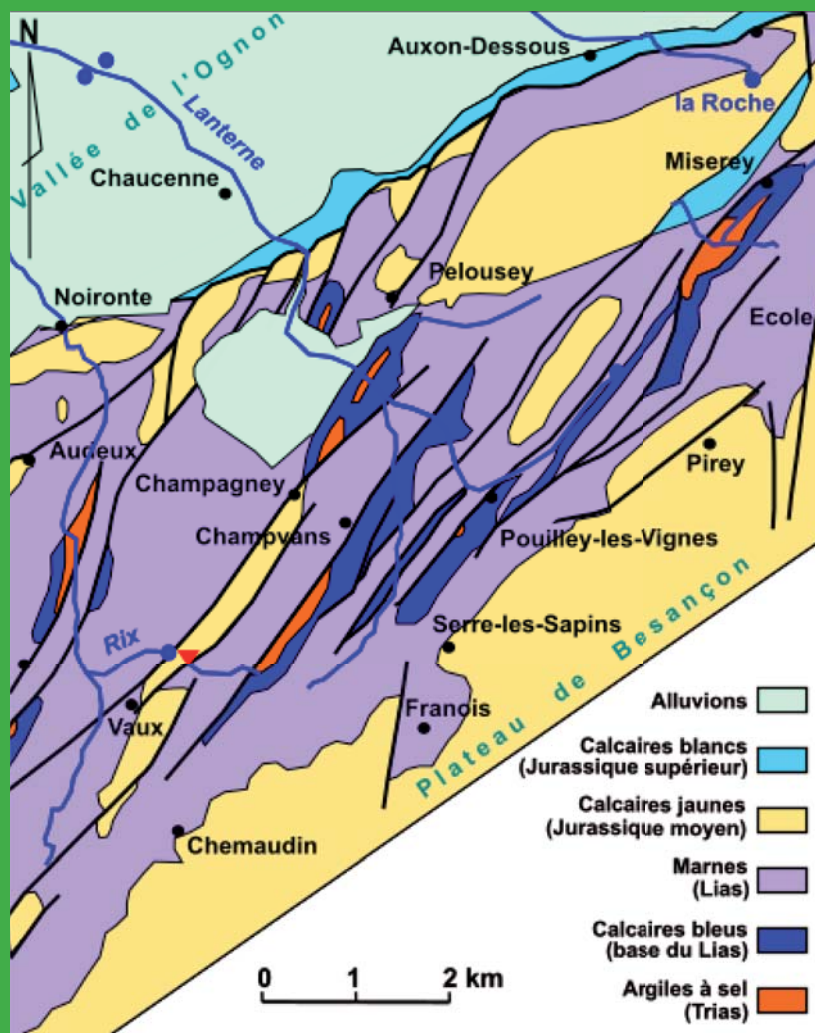
Figure 1 : Carte géologique des Avant-Monts, entre Audeux et École.
