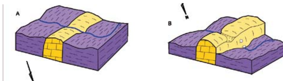
Fig. 7 : Traversée de la barre calcaire des Cotards par le Rix au cours du temps.
