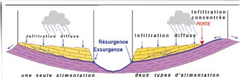
Fig. 1 : Les deux voies de l'infiltration
