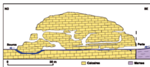
Fig. 4 : La grotte de Vaux-les-Prés.
