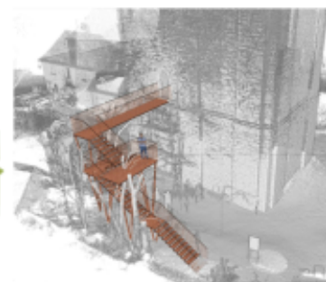
Accès à la porte d'entrée par un escalier métallique et une passerelle
