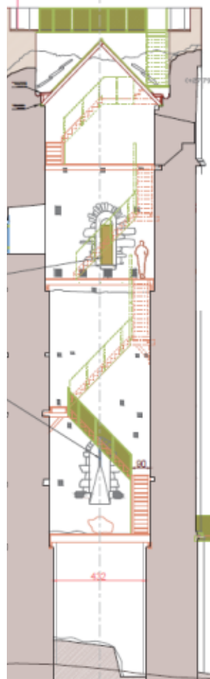
Accès à la porte d'entrée par un escalier métallique et une passerelle
