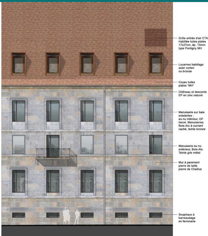
Illustration du dessin et de la matérialité des façades
