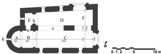
Fig. 1a - Plan en élévation de l'église romane du XIIe siècle
