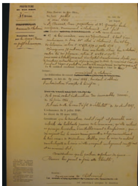
Burrus
