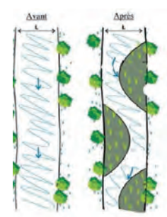
1 - Recharge granulométrique sous forme de banquette - Schéma de principe
